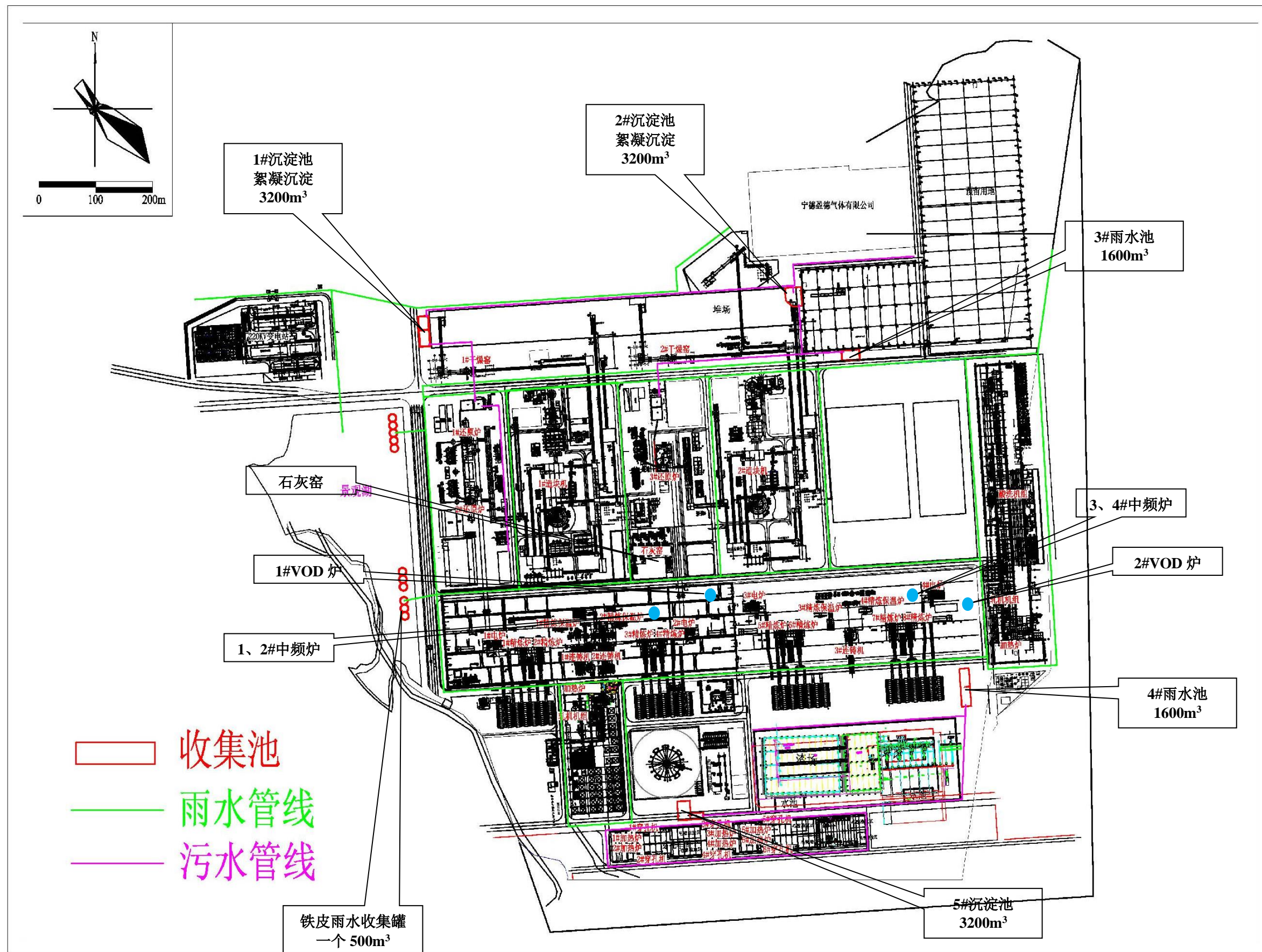
图 3.2-1 全厂雨污管线图
