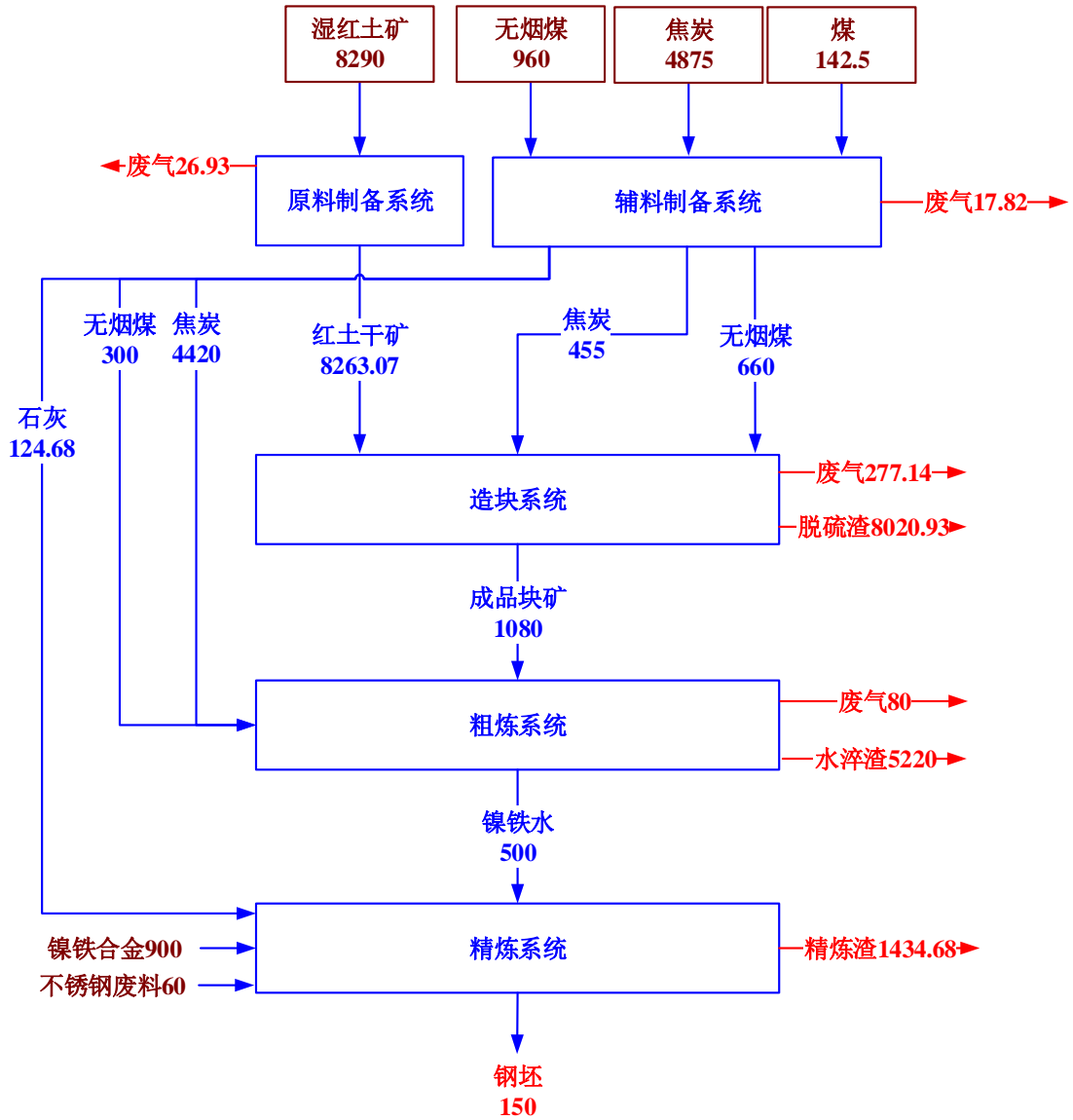
图 3.3-5 硫元素平衡图 (单位: t/a)
