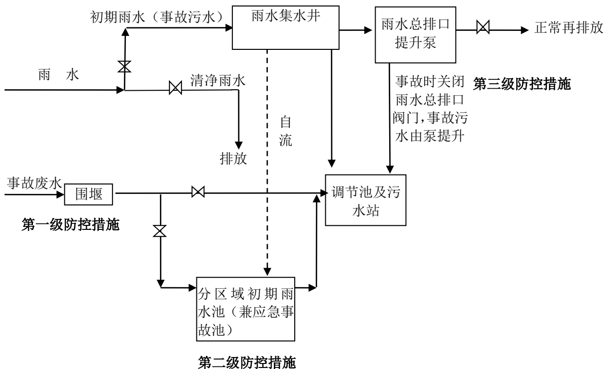
图 6.5-2 环境风险三级防控及切换系统
