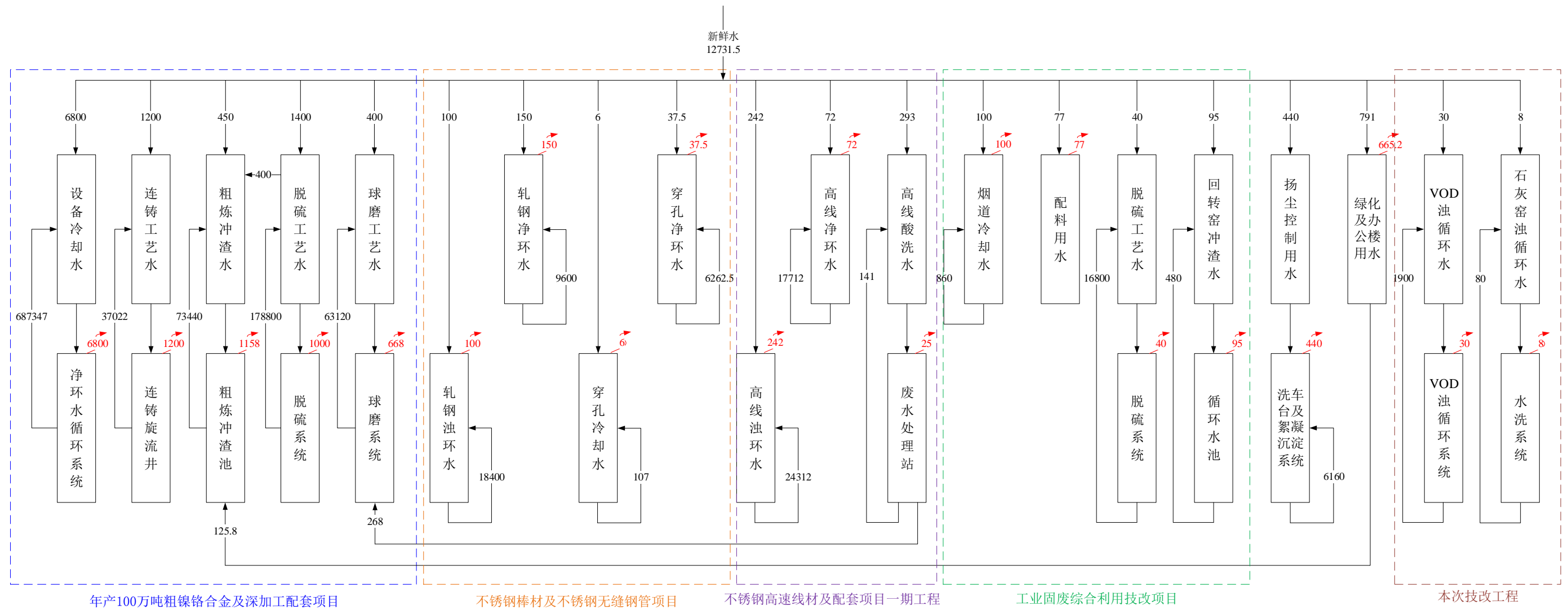
图 3.3-6 技改完成后全厂水平衡图 单位: t/d
