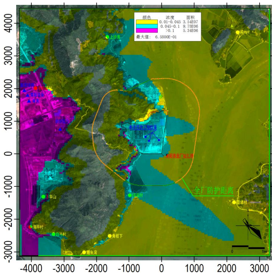
图 5.1-3 本项目技改后叠加现状浓度 100%保证率镍日均浓度预测值等值线图 \mu\text{g}/\text{m}^3
