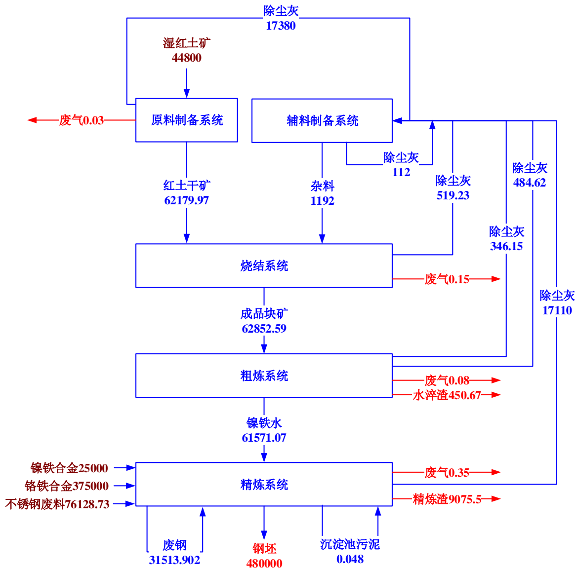
图 3.3-4 金属铬平衡图 (单位: t/a)
