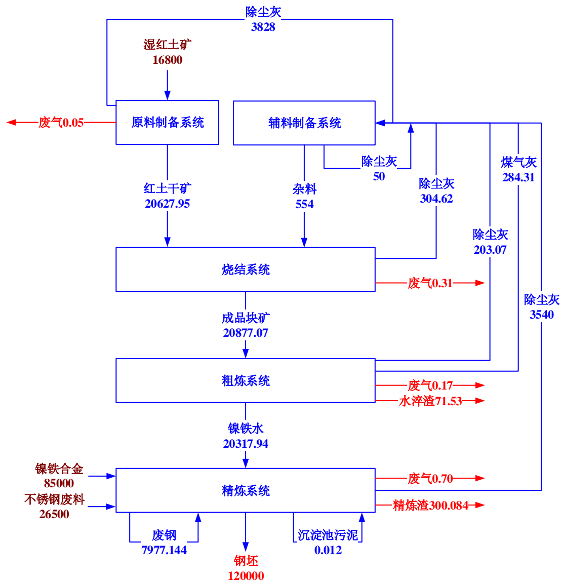
图 3.3-3 金属镍平衡图 (单位: t/a)
