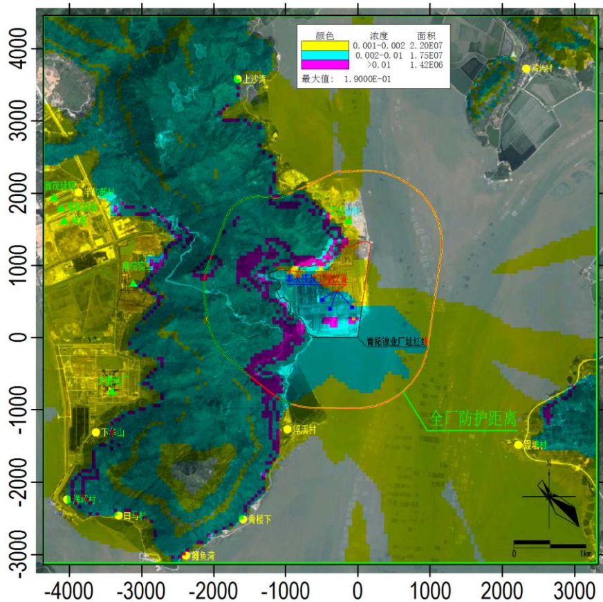
图 5.1-4 本项目技改后叠加现状浓度 100%保证率铬日均浓度预测值等值线图 \mu\text{g}/\text{m}^3
